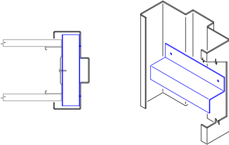
Welded Steel Stud Anchor (WSC)
